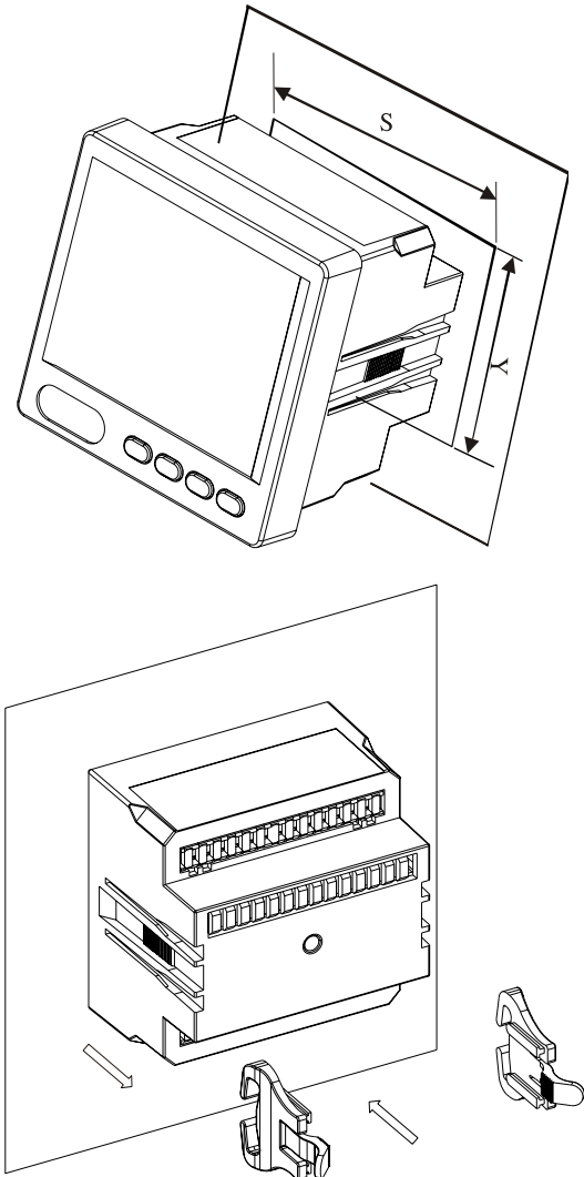
图 2 安装示意图
