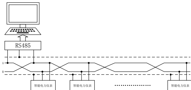
图11 T型网络连接方式
