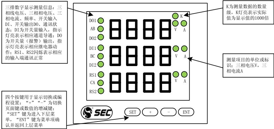
图10 面板说明与测量信息显示
