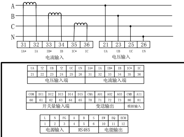
图4 72×72多功能电力仪表端子布置图1
