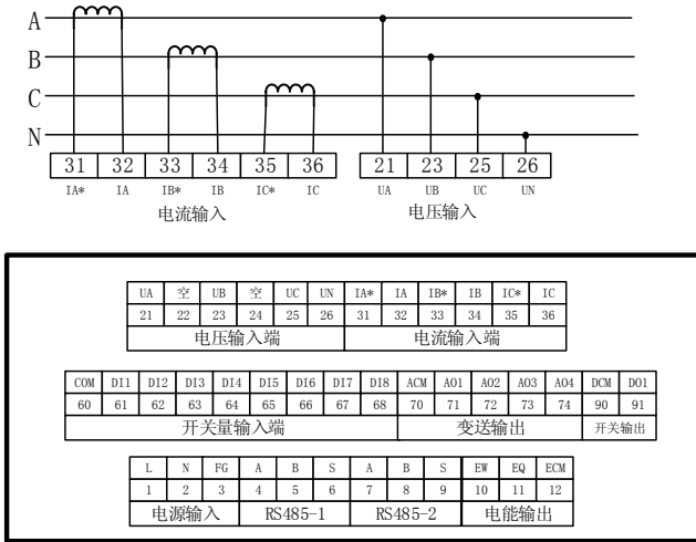
图3 96×96多功能电力仪表端子布置图1
