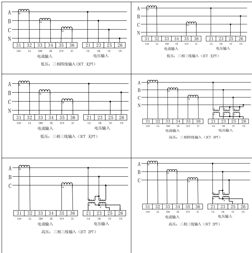
图 7 典型输入信号接线图
