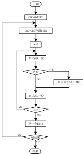
图13 CRC16校验
