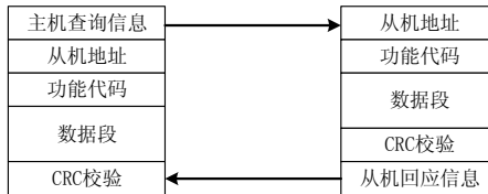
图12 主机与从机之间的通讯
